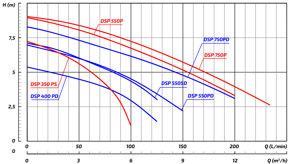
CURVA DE PERFORMANCE HIDRÁULICA A 50 HZ Alturas expresadas en m.c.a
